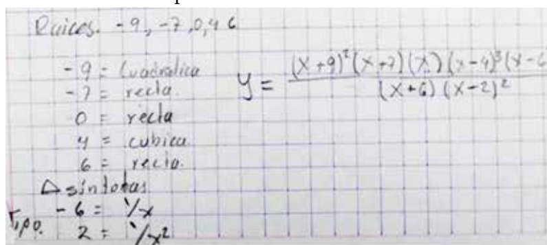
Figura 11. Propuesta de expresiones algebraicas para funciones racionales
